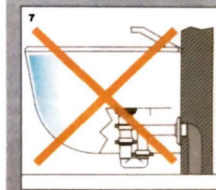
7. ESEMPIO di installazione scorretta.
