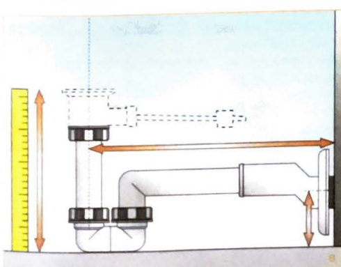
4. LA POSSIBILITÀ di rotazione di 3,5 cm ne permette un agevole inserimento nel foro di scarico.
