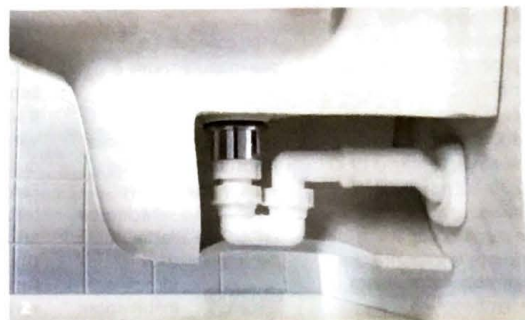
2. ESEMPIO di installazione del sifone eccentrico su un bidet.
