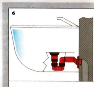
6. ESEMPIO di installazione corretta.
