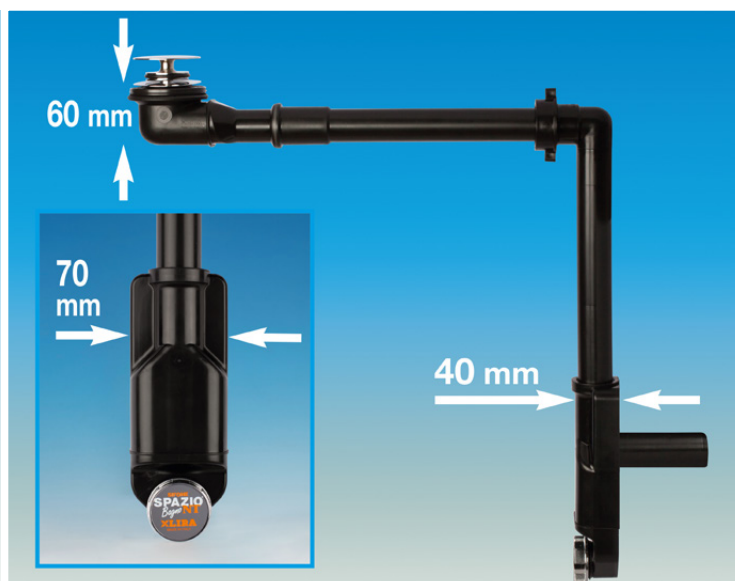
SOPRA Dimensioni Sifone e Piletta
